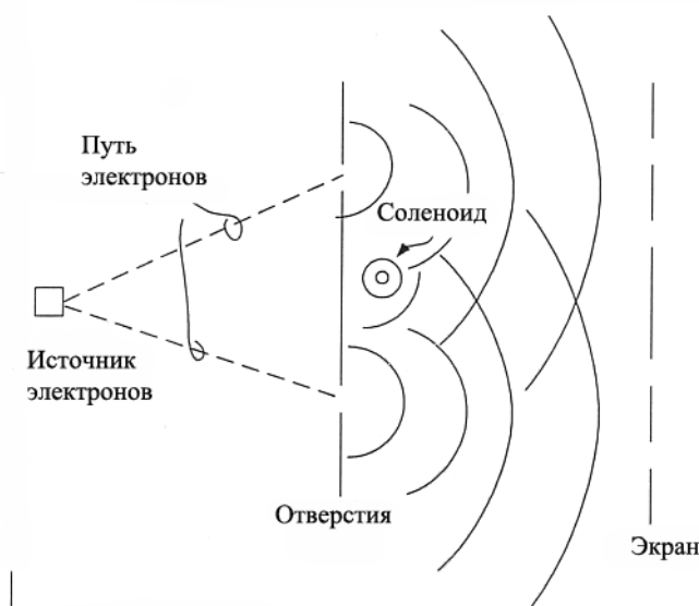
Рис. 3: Эффект Ахаронова Бома
